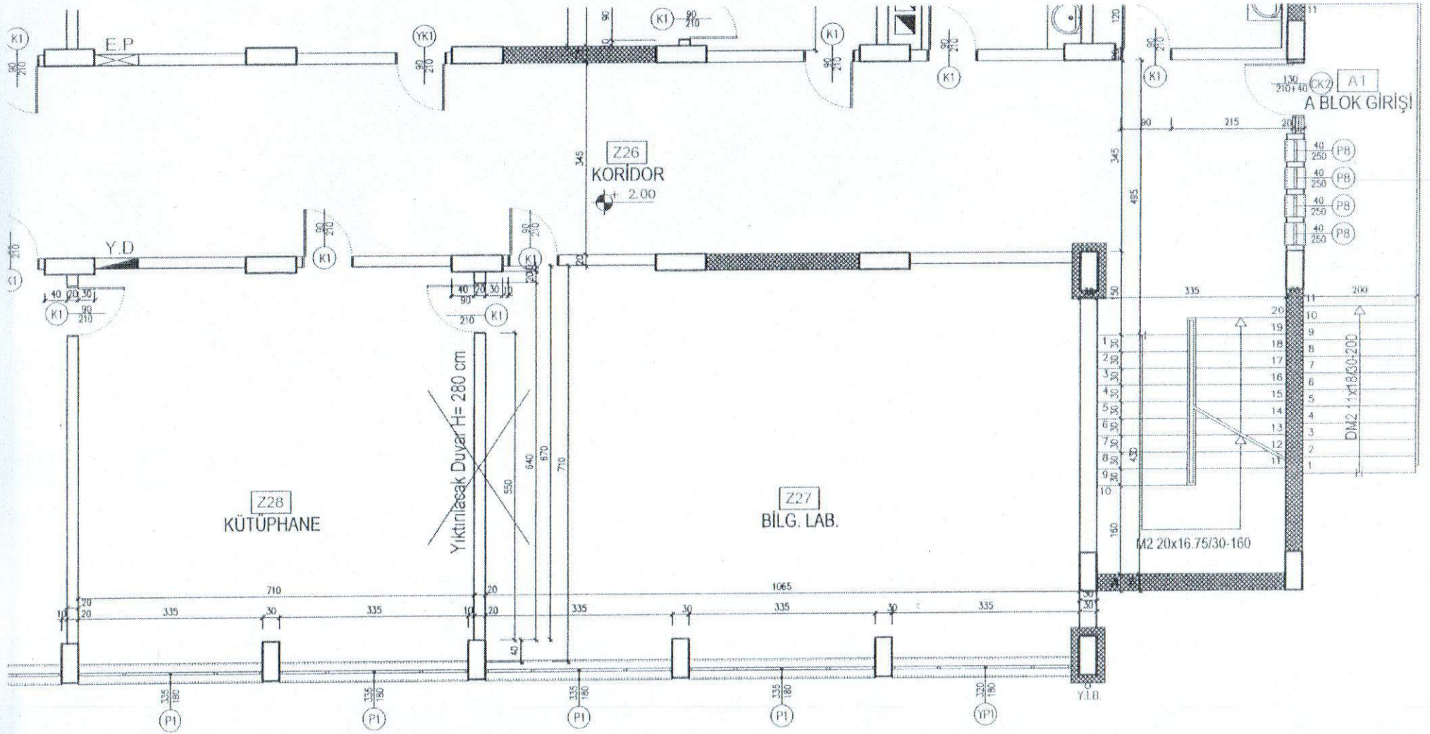
ZEMİN KAT PLANI - TADILAT ÖNCESİ DURUM KROKİSİ
